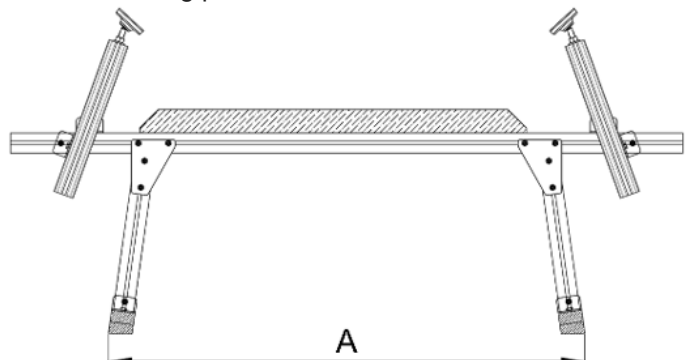
Max belastning per bock. Bestäms av benavståndet A
